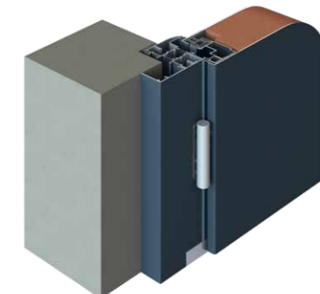
POSE EN FEUILLURE Dormant large sans aile + compensateur de feuillure
