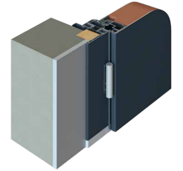
POSE EN RENOVATION SUR DORMANT EXISTANT Dormant avec aile de 60 mm + cornière de finition extérieure
