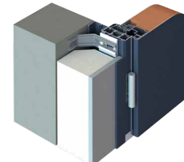
POSE EN APPLIQUE Dormant intermédiaire sans aile + tapée de doublage
