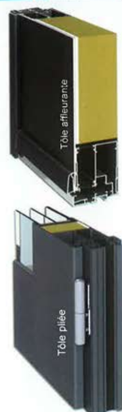
Coupes de Portabloc, gamme d'ouvrants monobloc en aluminium d'Euradif.
