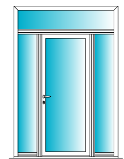
CAS 6 Imposte et tierces identiques
