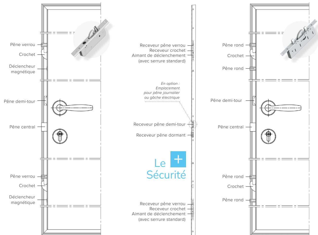
1 SERRURE AUTOMATIQUE 5 points avec 2 crochets et 2 pènes verrous
